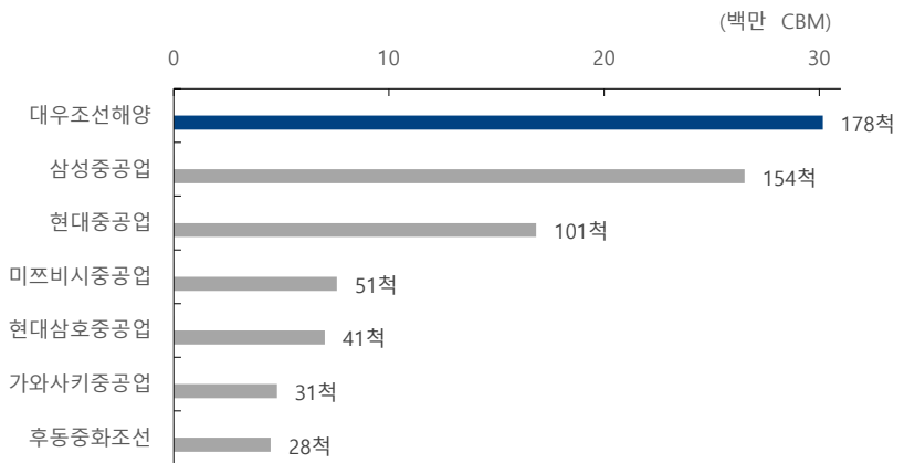
그림4. LNG 운반선(+40K CBM) 인도 실적 ('22.2 월 기준)
