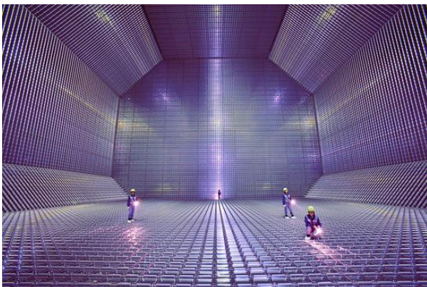
그림6. 작업 막바지 단계의 LNG 화물창 내부
